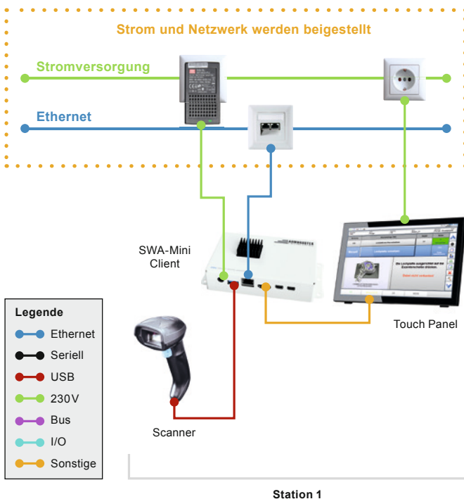
Geräteplan zur Anbringung des SWA-Mini Clients
